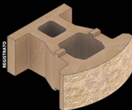
Tutti i blocchi sono con finitura splittata faccia a vista
